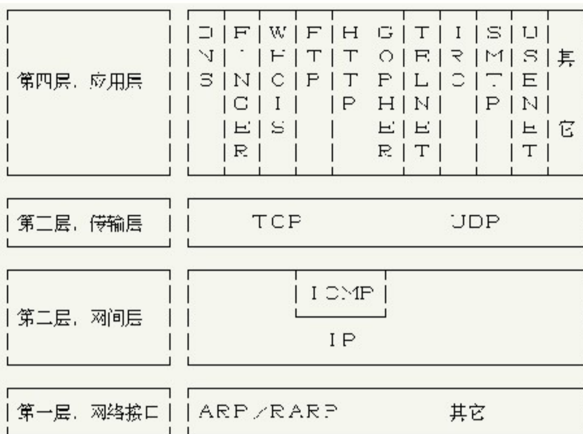
TCP/IP 四层网络模型
